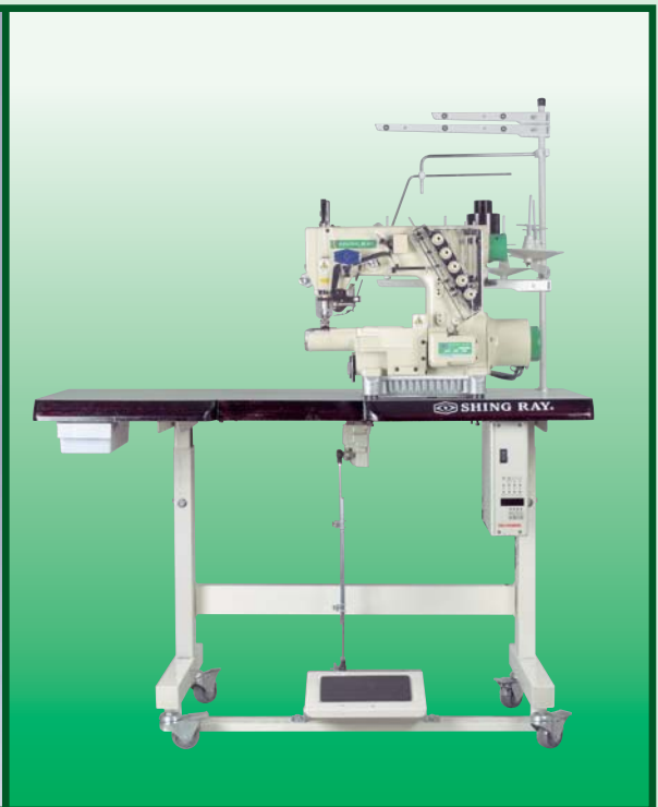
直驅、外接下主軸心式微型伺服馬達
